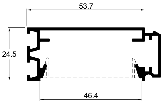
VL039 0,658 kg/m Arremate de folha
