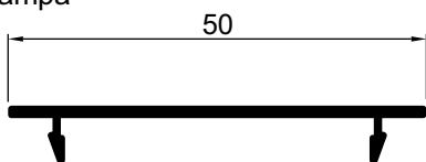
UN217 0,243 kg/m Tampa
