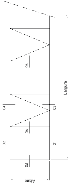
ELEVAÇÃO VISTA EXTERNA
