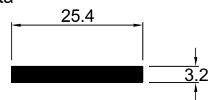
BC025 0,219 kg/m Barra chata
