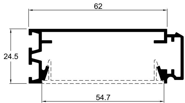
LC036 0,688 kg/m Arremate de folha
