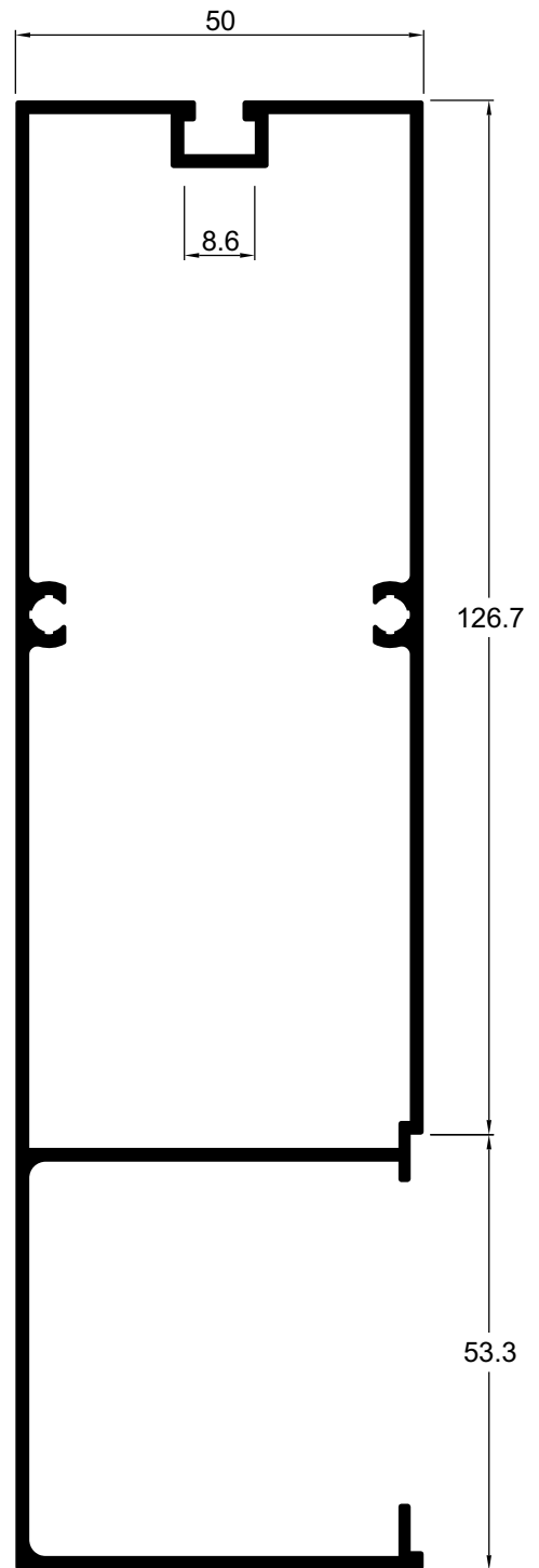
LU039 2,315 kg/m Brise
