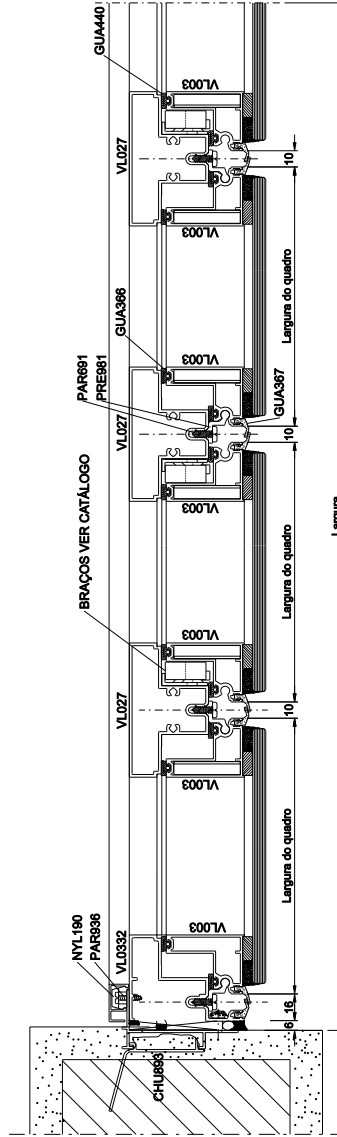
Corte 08
