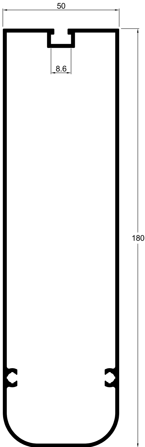
LU038 2,226 kg/m Brise
