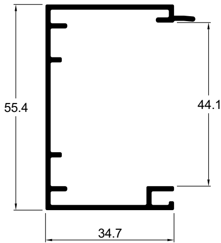
LU065 0,903 kg/m Travessa
