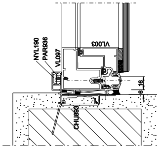
Corte 05 (Opção com perfil VL097)
