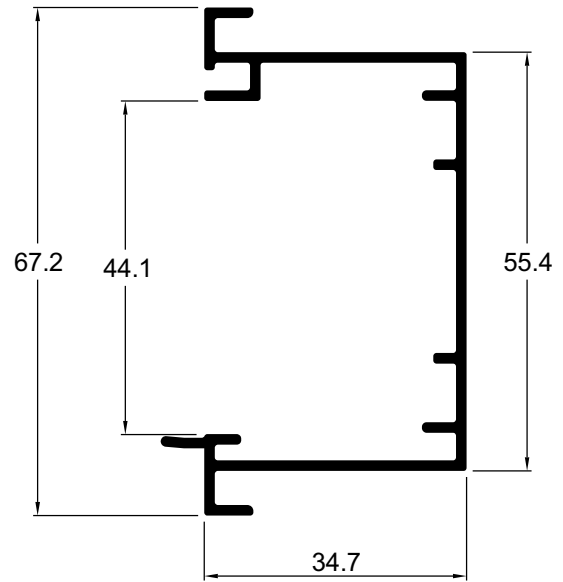
LU066 0,494 kg/m Tampa
