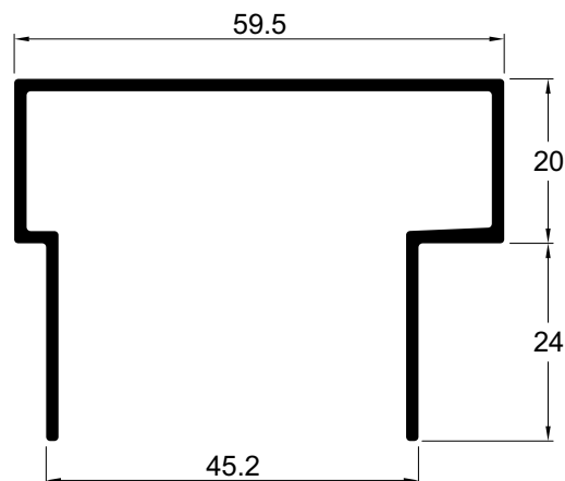
CM234 0,345 Kg/m Complemento inferior da calha com 50 mm
