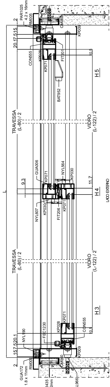
Janela de correr 2 folhas c/ fecho no marco
