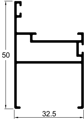
KP067 0,709 kg/m Folha montante e travessa
