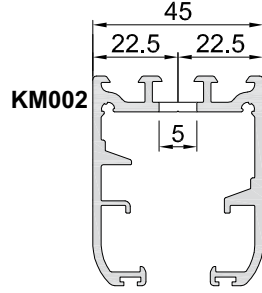
Corte AA
